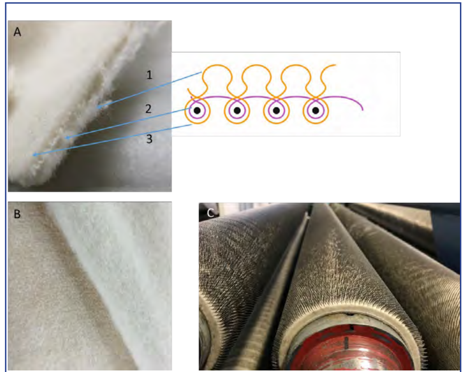
Abb. 1: Schichtartiger Aufbau der Flächenkonstruktion für einen Fleecestoff. Garnverteilung innerhalb der Umkehrplattierung: Bild A, 1+3=Polfaden, außen auf rechter und linker Wareseite, hier beidseitig geraut, Bild B: Grundfaden (innenliegend), im Rauprozess weitgehend unbeschadet), Beispiel für ein Fleece material, Darstellung der Rauwalzen (C) Abbildungen: Hochschule Niederrhein
